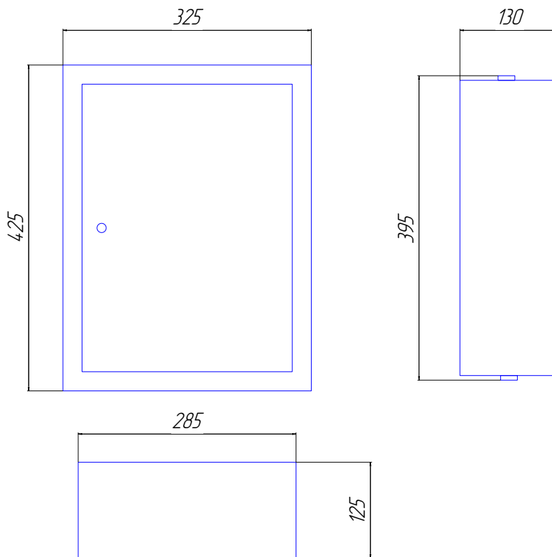
Рис. 1 Габаритные размеры.
